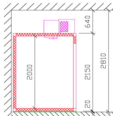
Nákres MINI 3000-N s jednotkou A
