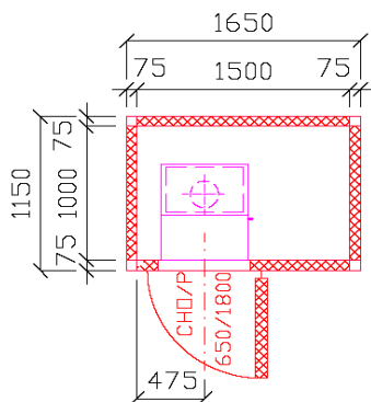
Nákres MINI 3000-N s jednotkou A
